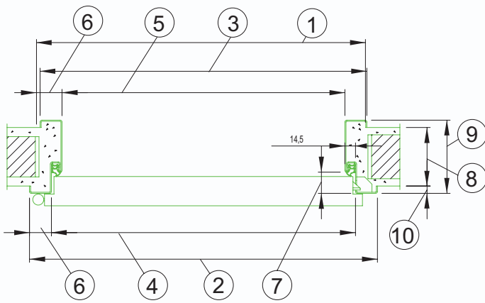
Horizontalschnitt
